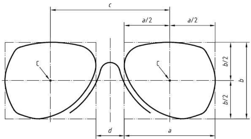
그림 1 선글라스 치수의 측정 (전면부)
