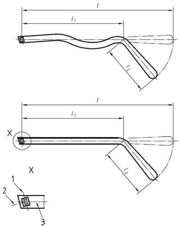
그림 2 선글라스 치수의 측정 (다리)
